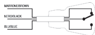
SCHEMA COLLEGAMENTI CONNECTION DIAGRAM SCHÉMA DE CONNEXION
